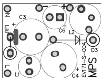
Top layer
