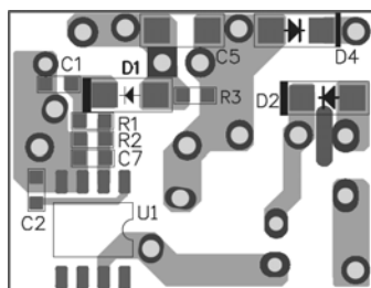
Bottom layer
