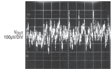
C OUT = 10µF I L = 100mA 1ms/DIV 1761 G46
