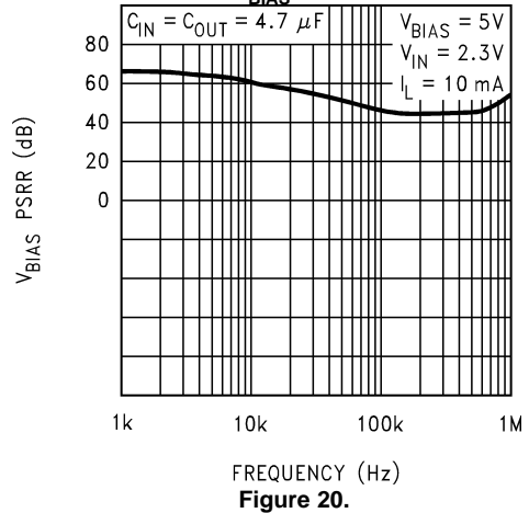
VBIAS PSRR
