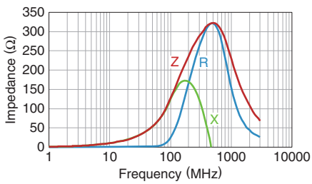
MMZ1608Q471BTD25
