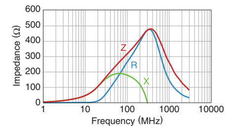
MMZ1608Y301BTD25
