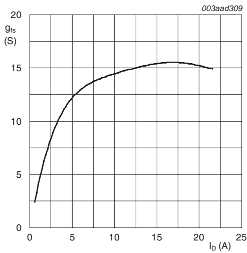
T_j = 25\text{ °C} ; V_{DS} = 15\text{ V}
