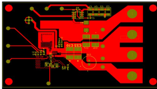
Figure 17. Bottom Layer
