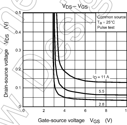
Fig. 8.4 V_{DS} - V_{GS}
