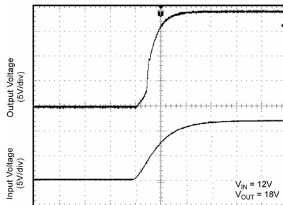
Input Turn-On
