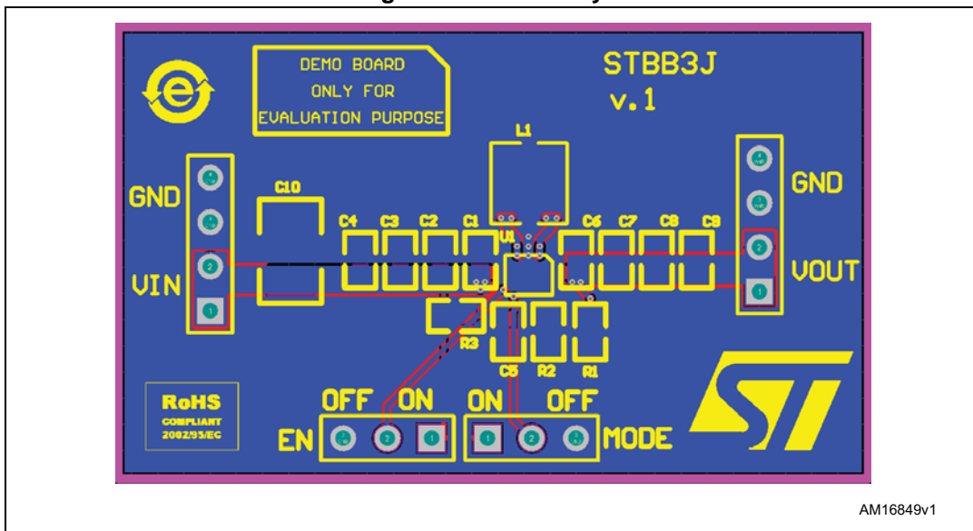
Figure 34. Bottom layer
