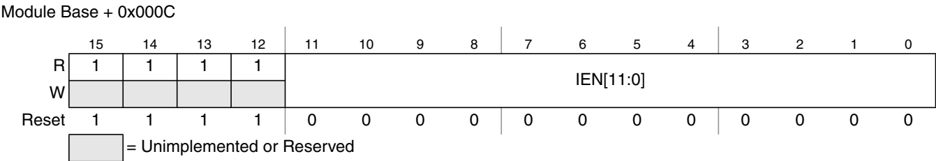
Figure 14-12. ATD Input Enable Register (ATDDIEN)
