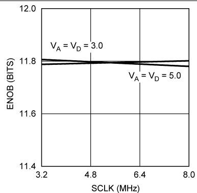
Figure 24. ENOB vs SCLK
