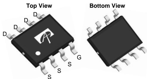
SOIC-8
