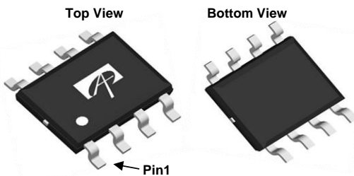
SOIC-8
