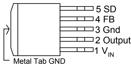
TO263-5L
