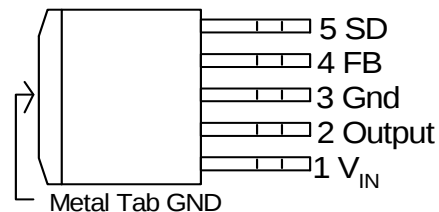
TO263-5
