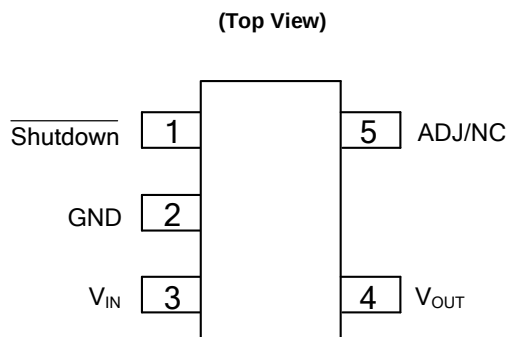
SOT-23-5
