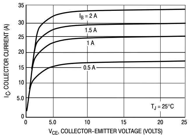
NPN NJL21194
