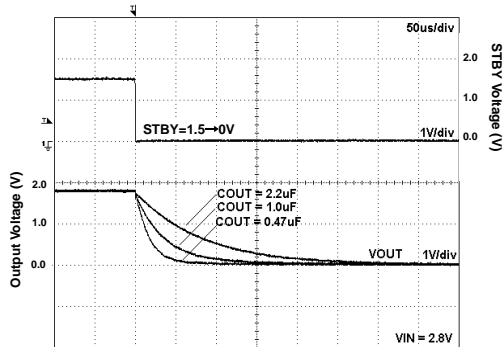
Fig 26. Discharge Time
