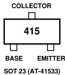
SOT 23 (AT-41533)
