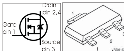
PG-SOT223
