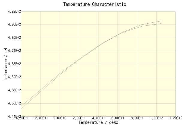
CLF12555T-471M-CA(DC = 0A)
