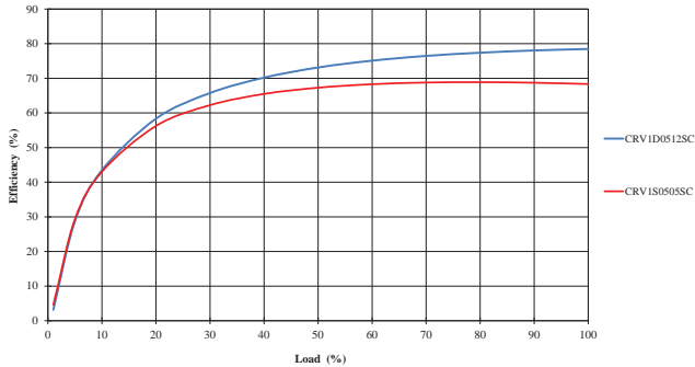
5V Inputs
