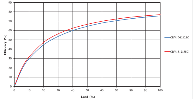
12V Inputs
