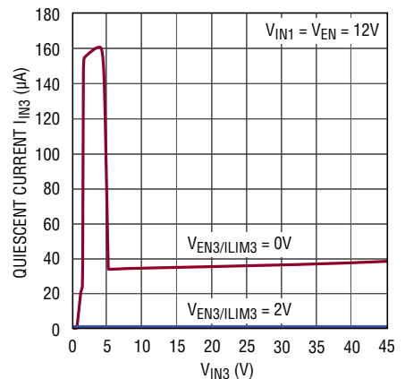
LDOs: 5V Quiescent Current IN3
