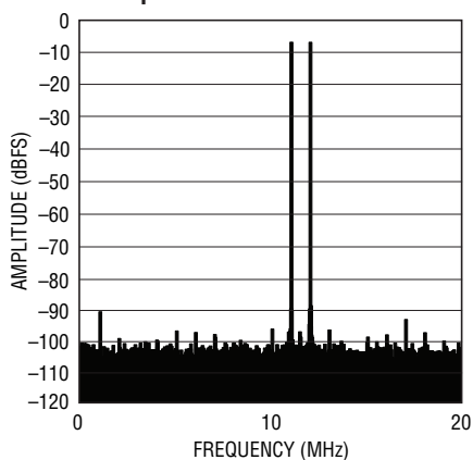
LTC2264-14: 8k Point 2-Tone FFT, f_{IN} = 68\text{MHz} , 69\text{MHz} , -1\text{dBFS} , 40\text{Mps}
