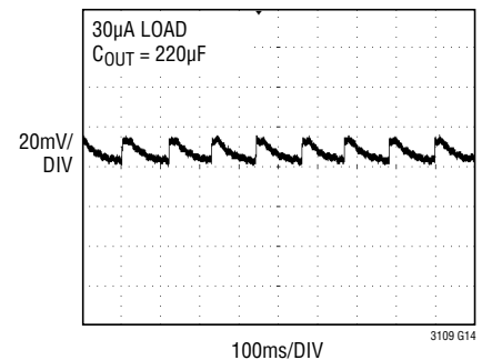
V_{OUT} Ripple
