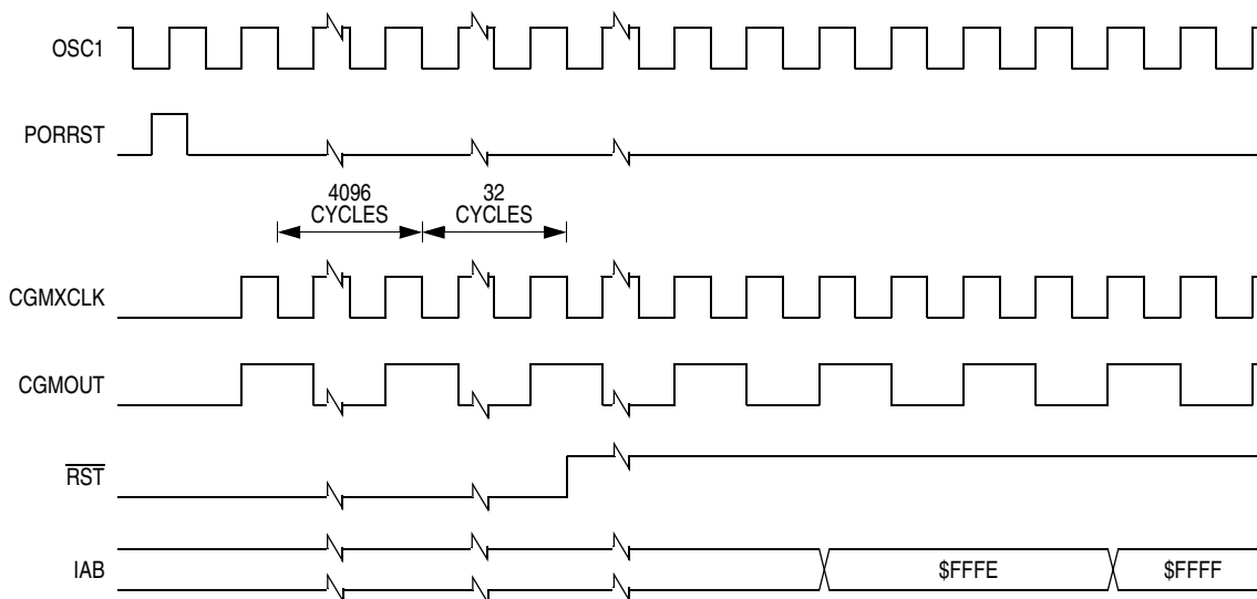
Figure 16-7. POR Recovery
