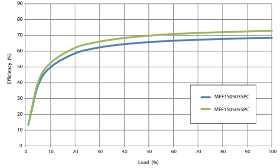
5V Input
