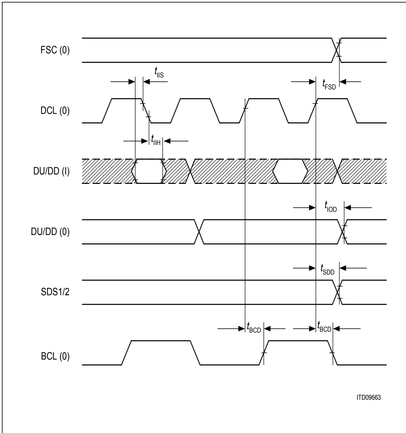
Figure 79 IOM ® Timing
