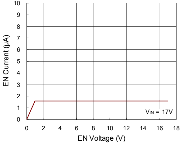
EN Current vs. EN Voltage
