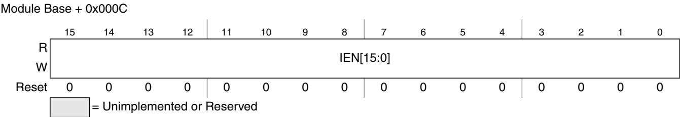
Figure 15-12. ATD Input Enable Register (ATDDIEN)
