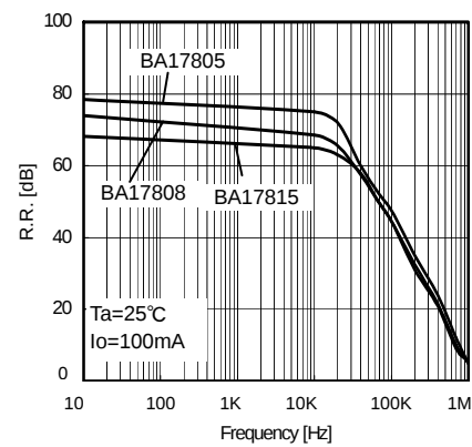
Fig.21 リップル除去率
