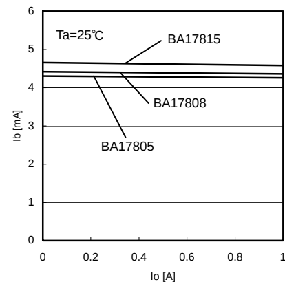
Fig.24 出力電流－バイアス電流
