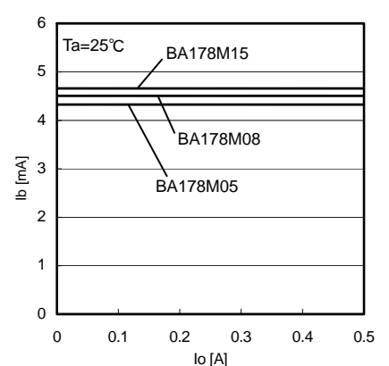
Fig.12 出力電流-バイアス電流
