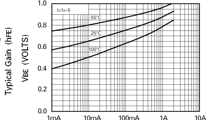
VBE(SAT) vs IC
