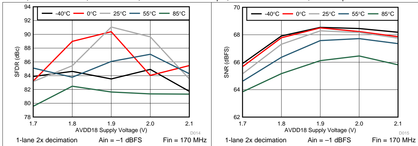
Figure 18. SFDR vs. AVDD18
