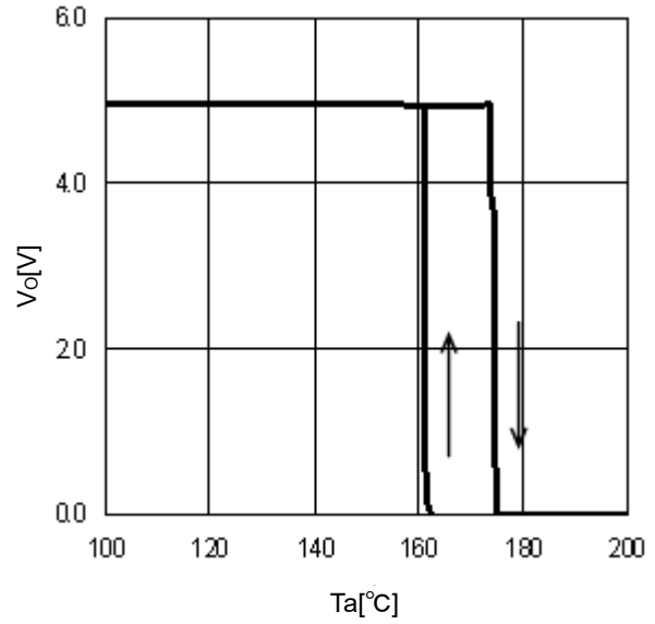
Figure 28. TSD (Io=0mA)
