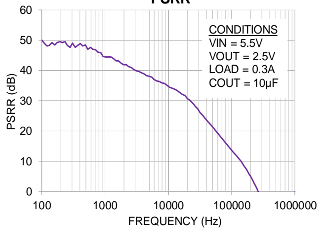
PSRR
