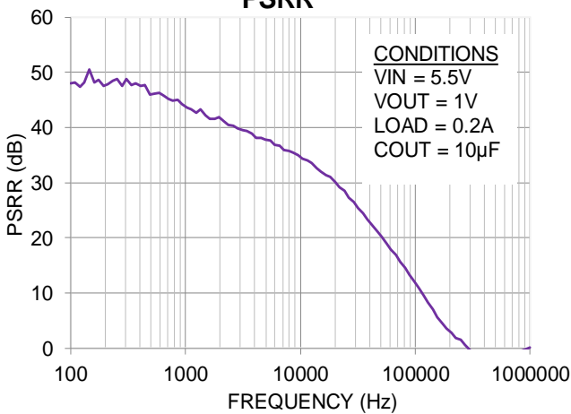
PSRR
