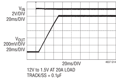
Turn-On 20A Load
