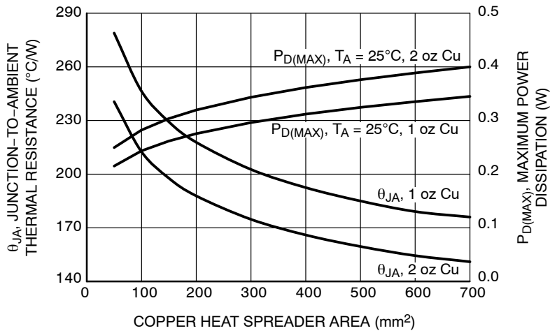
Figure 45. \theta_{JA} vs. Copper Area (uDFN4)
