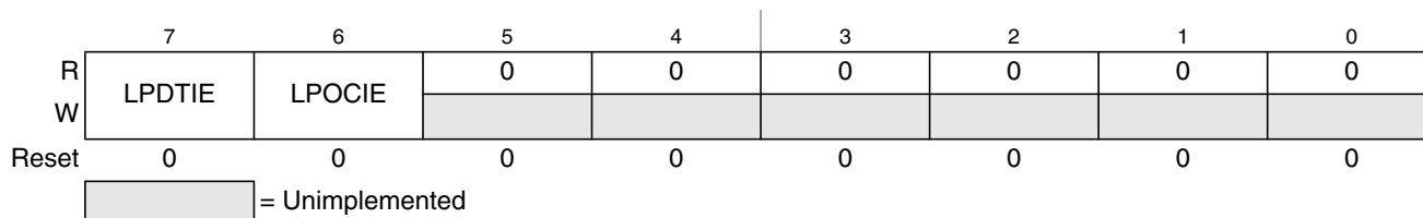
Figure 15-9. LIN Interrupt Enable Register (LPIE)
