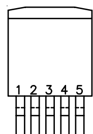
TO-263-5
