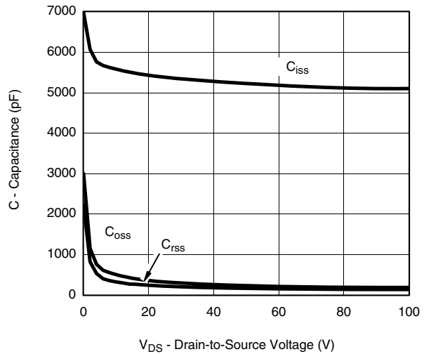
C_{iss} C_{oss} C_{rfs} Capacitance
