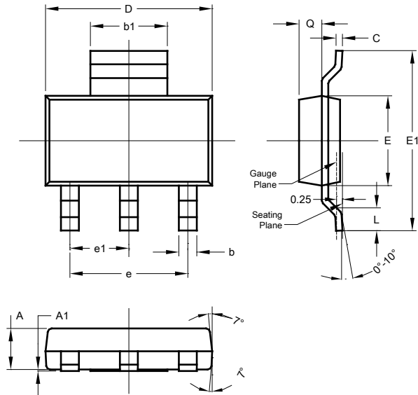
SOT223
