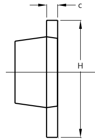
SOT89
