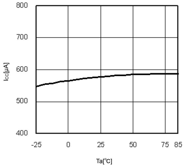
Fig.10 Ta-Icc
