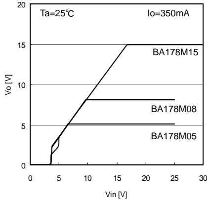
Fig.2 電源電圧-出力電圧 (Io=350mA)
