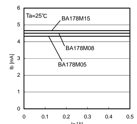
Fig.12 出力電流-バイアス電流
