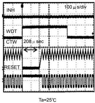
Fig.44 WDT Edge Pulse Width
