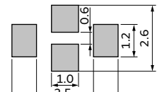
NFM31PC/31KC
