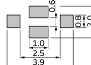
NFM3DCC/3DPC
