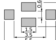
NFM41CC/41PC
