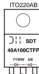
ITO220AB (Type HE)
