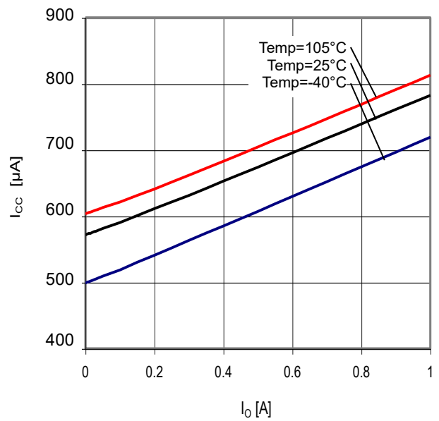
Fig.30 I_o-I_{cc}
