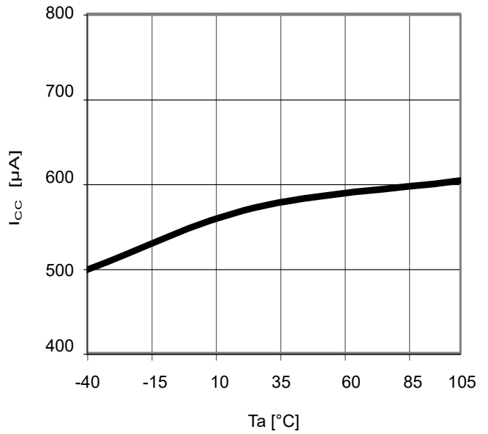
Fig.22 Ta-I cc
