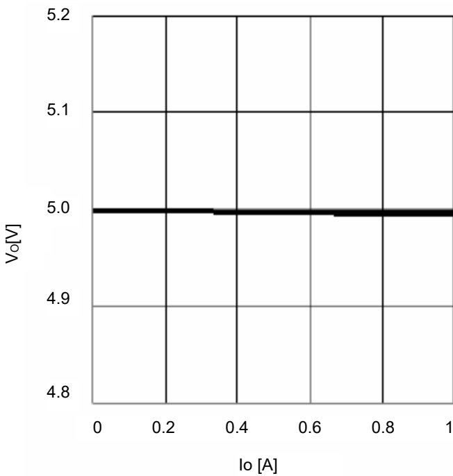
Fig.25 I_O - V_O
